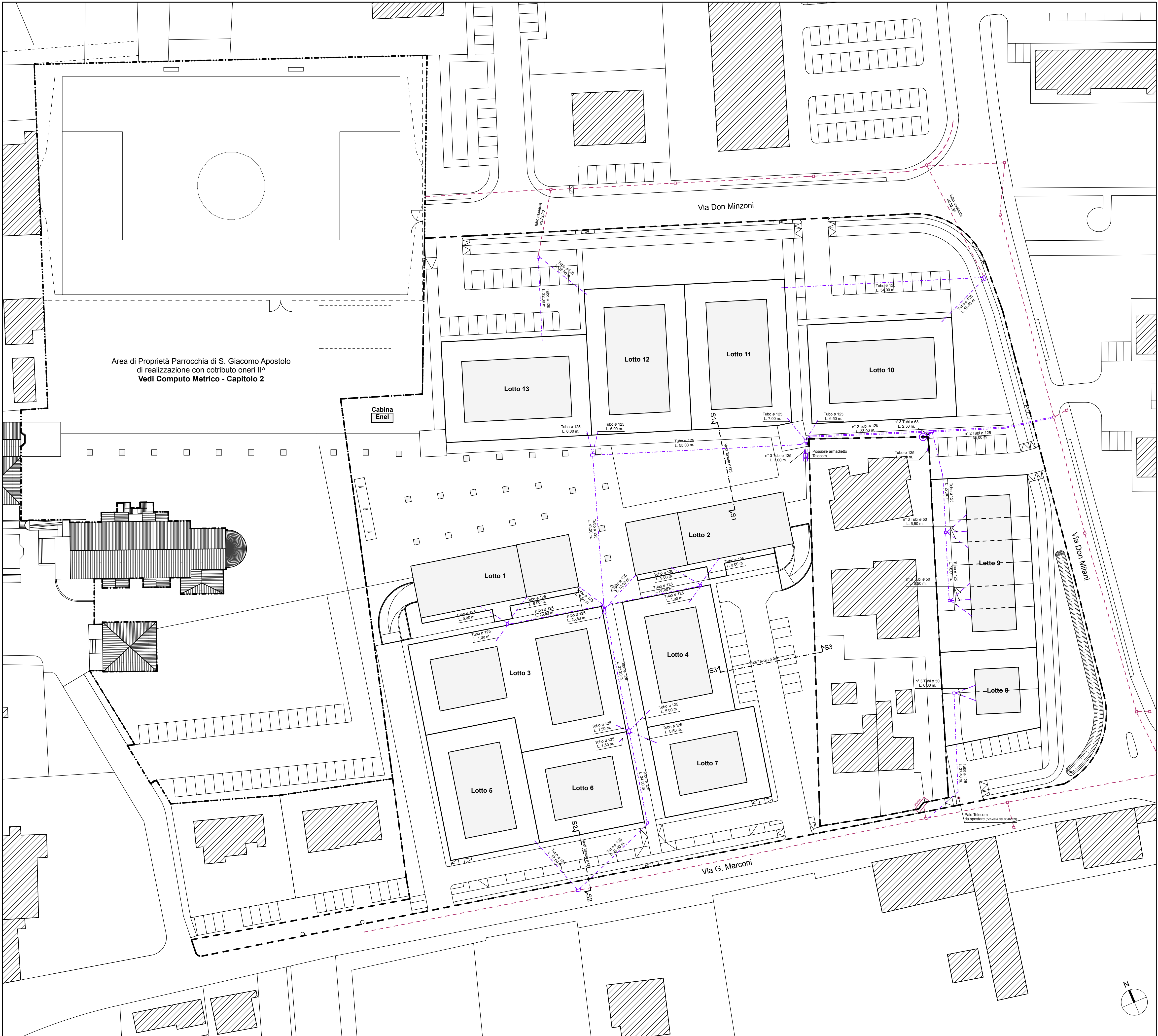
Planimetria con Rete Telecom di Progetto scala 1:500
